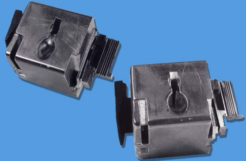
Spannen von Flugzeugturbinenschaufeln und Leitschaufeln mit MCP 137
